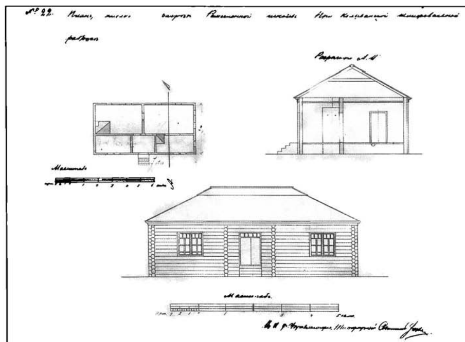
План, фасад и разрез ремесленной школы при Колыванской шиферной фабрике, б/д. ЦХАФ АК. Ф. 50. Оп. 11. Д. 118
